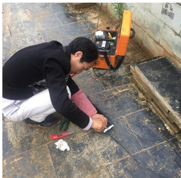
现场熔接光纤图 2
