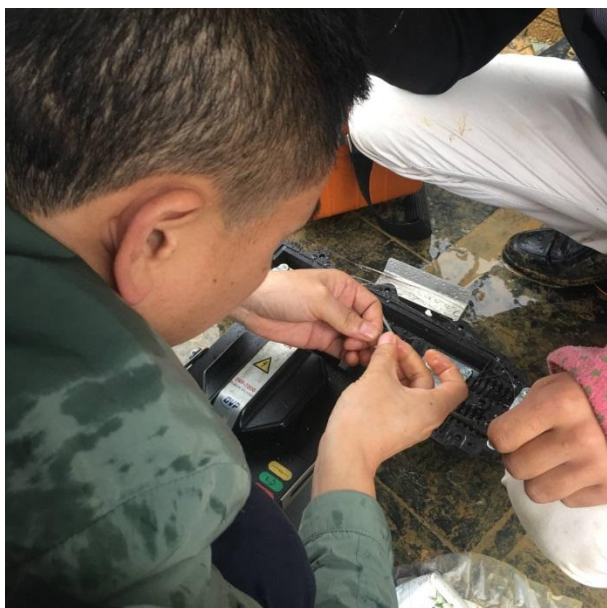
现场熔接光纤图 3
